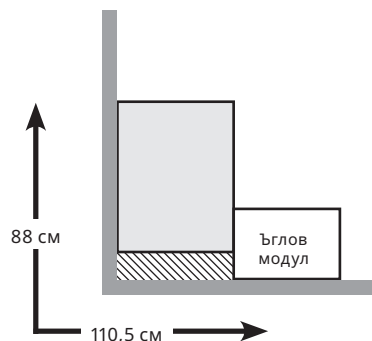
Ъглов модул с дълбочина 35 см в комбинация с рамка 75x58 см
