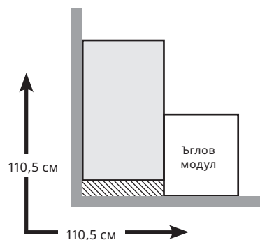
Ъглов модул с дълбочина 58 см в комбинация с рамка 100x58 см
