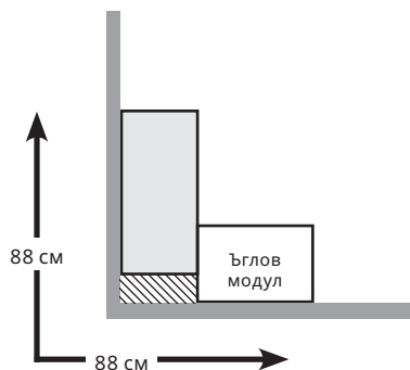
Ъглов модул с дълбочина 35 см в комбинация с рамка 75x35 см
